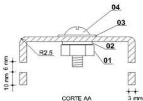
CORTE AA
